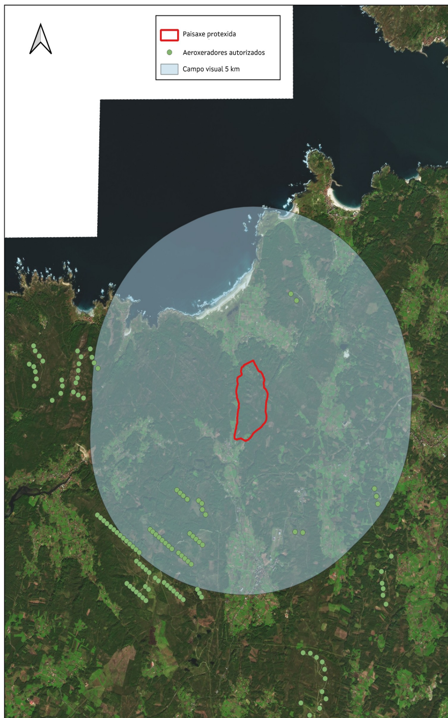
Mapa 5. Representación dos aeróxeradores localizados na contorna da paisaxe protexida; destácase o campo visual desde esta nun raio de 5 km.
