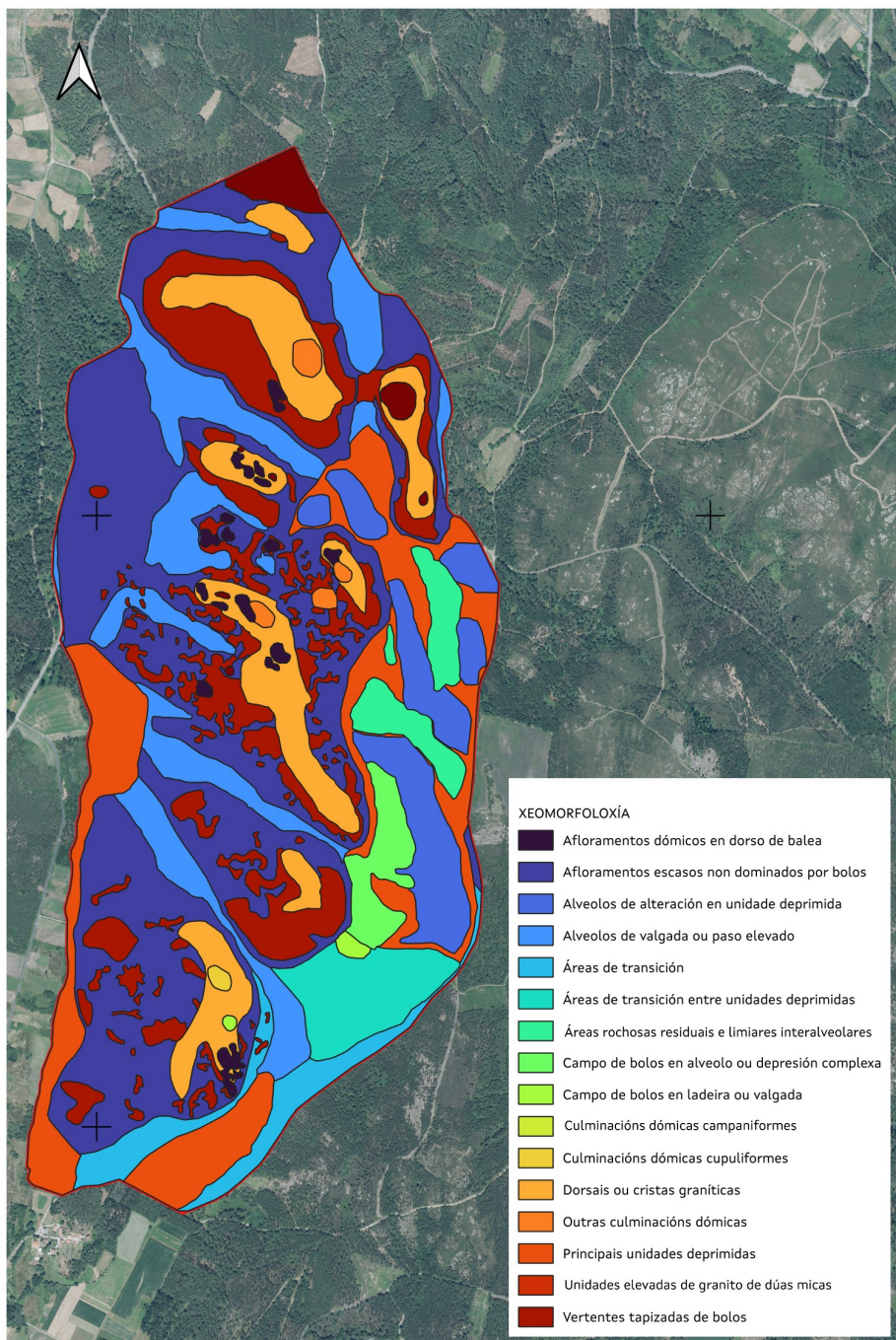
Mapa 2. Mapa xeomorfolóxico. Representación das diferentes unidades de superficie.
